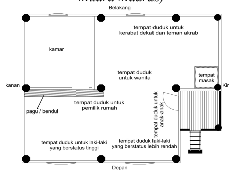
Gambar 8 : Sketsa Rumah Tradisional Desa Muara Madras Kecamatan Jangkat Kabupaten Merangin-tampak atas. (Sumber: ilustrasi Fori badria aswianto, sketsa Rumah Tradisional Desa Muara Madras)
