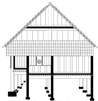
Gambar 7 : Sketsa Rumah Tradisional Desa Muara Madras Kecamatan Jangkat Kabupaten Merangin-tampak samping kanan. (Sumber: ilustrasi Fori badria aswianto sketsa Rumah Tradisional Desa Muara Madras)
