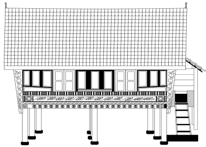
Gambar 6 : Sketsa Rumah Tradisional Desa Muara Madras Kecamatan Jangkat Kabupaten Merangin-tampak samping kiri. (Sumber :ilustrasi Fori badria aswianto sketsa Rumah Tradisional Desa Muara Madras)
