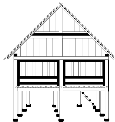
Gambar 5 : SketsaRumah Tradisional Desa Muara Madras Kecamatan Jangkat Kabupaten Merangin-Tampak depan. (Sumber: ilustrasi Fori badria aswianto, sketsa Rumah Tradisional Desa Muara Madras)
